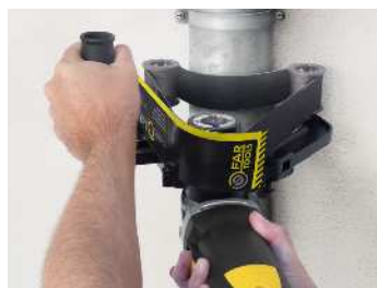
Carter pour aspiration des poussières Housing for dust extraction
