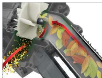
Fonction aspirateur / broyeur Vacuum / Crusher function
